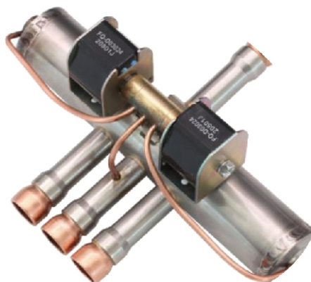
图4-20 四通阀
